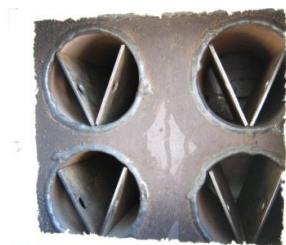
Рисунок 3 – Установка турбулизаторов
